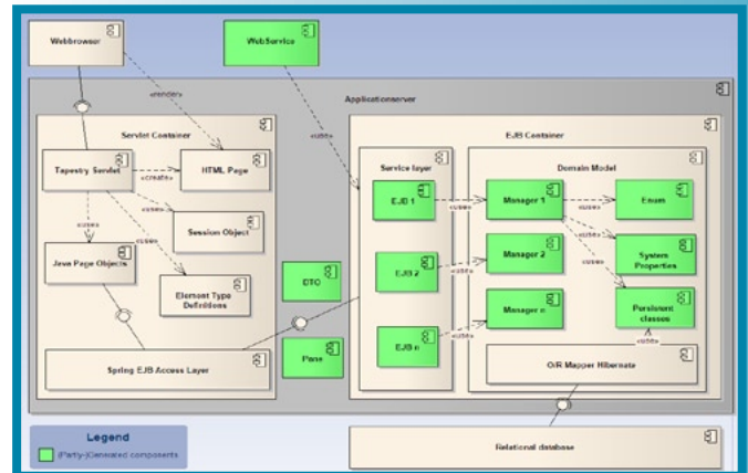
Abb. 7: DTC-Architektur mit Kennzeichnung der (teil-)generierten Komponenten
