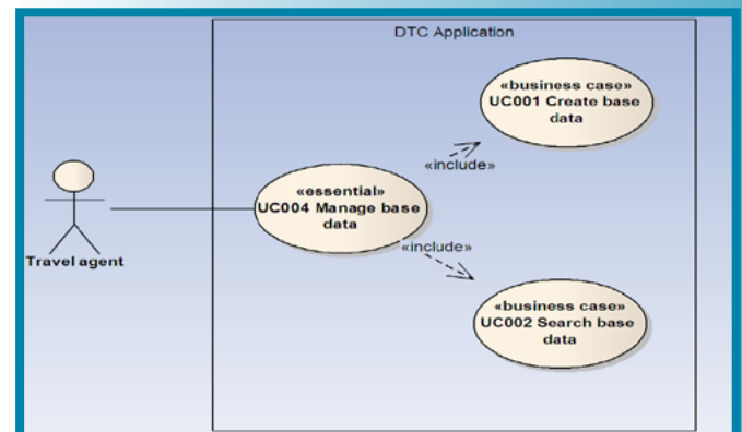
Abb. 3: Use-Case-Modellierung
